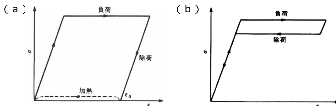
図1 形状記憶合金の応力ひずみ線図 (1) (a) 形状記憶効果 (b) 超弾性
