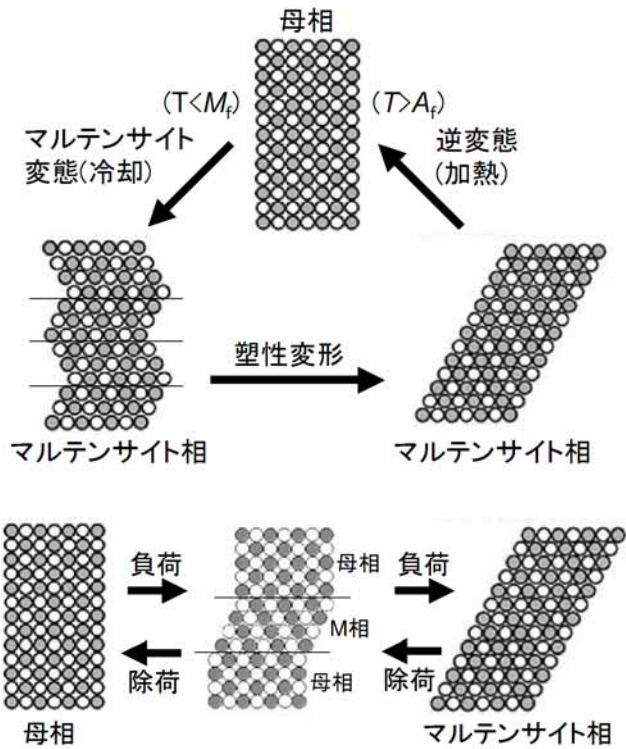
図3 形状記憶効果と超弾性の機構の模式図
