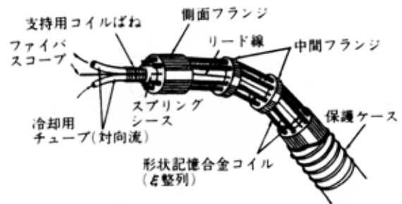
図2 内視鏡への利用 (2)
